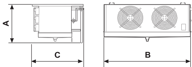
Evaporadores cúbicos
